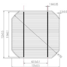
Monokrystalický článek s hustou sítí sběrných kontaktů
